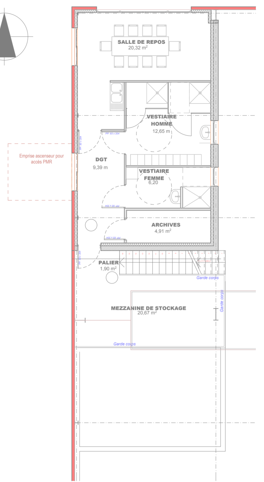
VUE EN PLAN NIVEAU R+1
